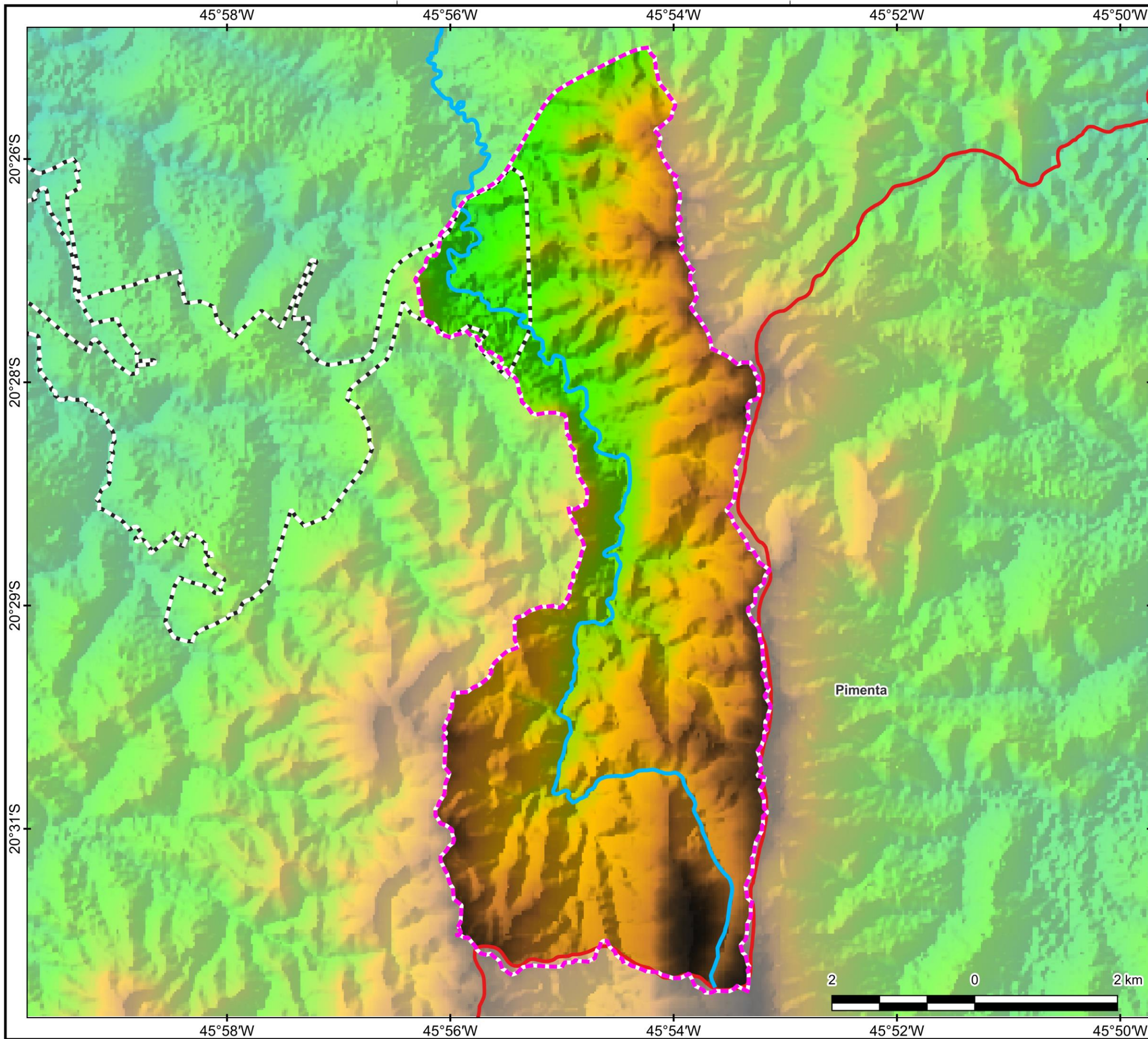
Mapa 5 - Hipsometria da área em estudo.
