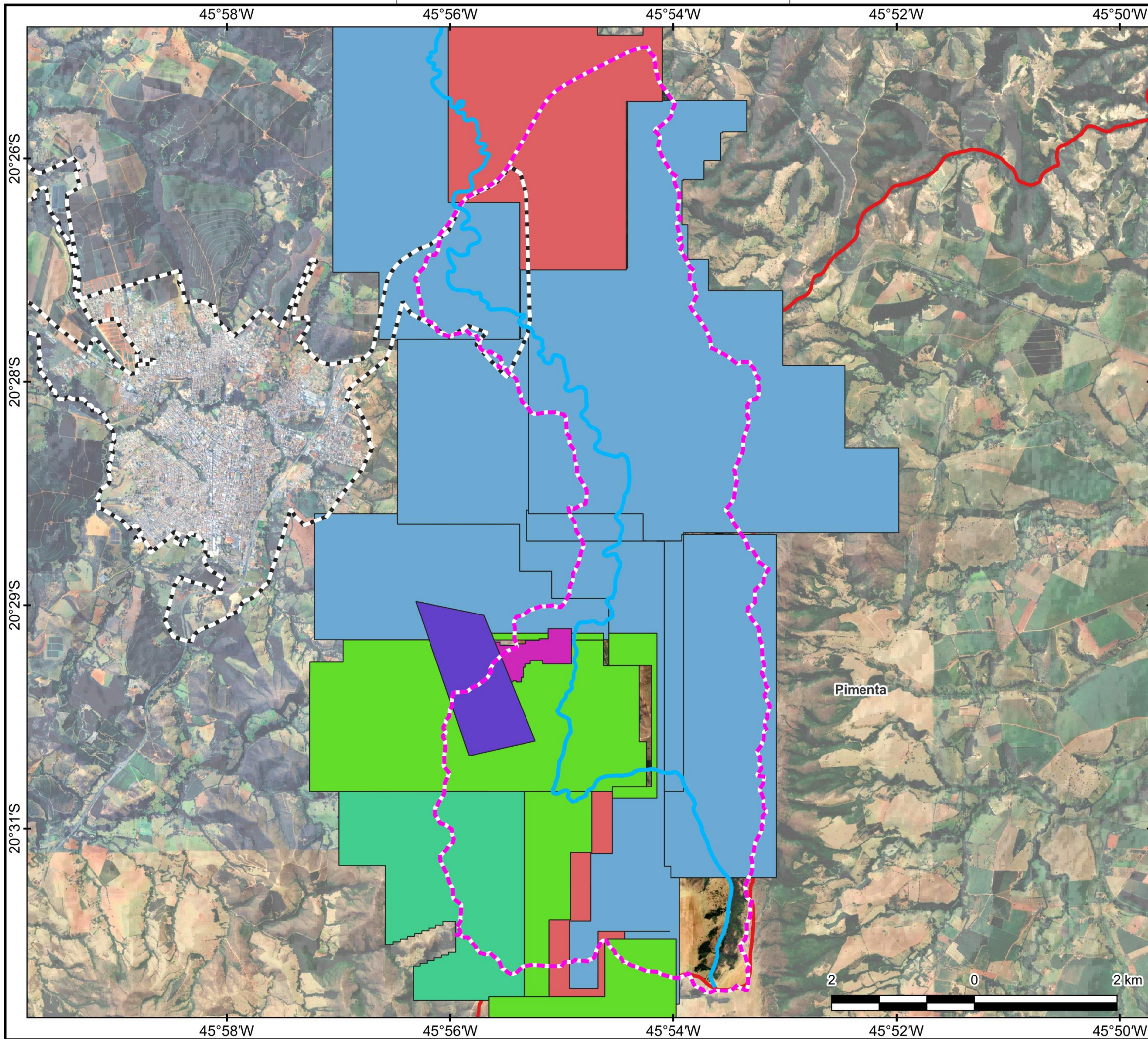
Mapa 20 - Processos minerários na área em estudo.
