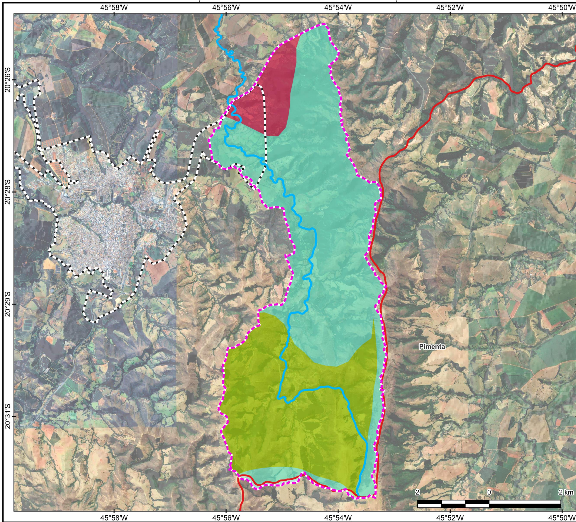
Mapa 8 - Pedologia da área em estudo.
