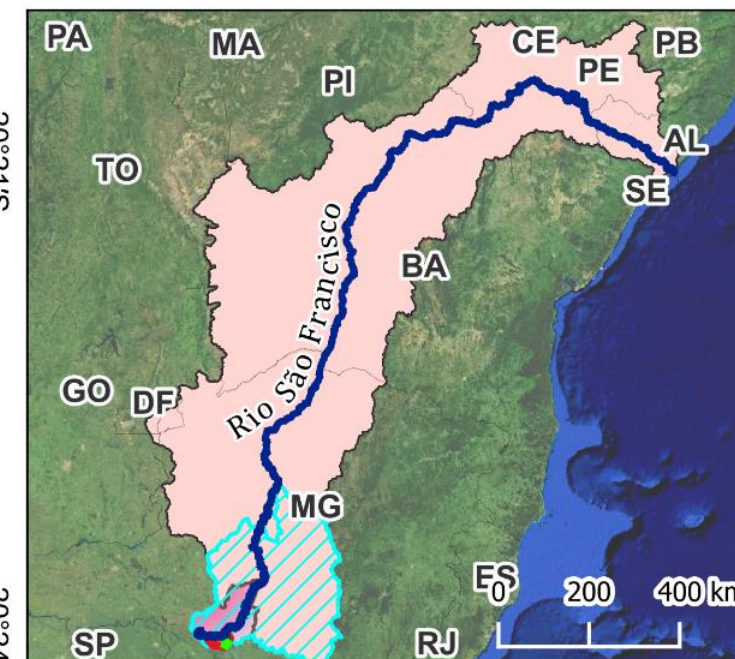
Mapa 10 - Hidrografia da área em estudo.
